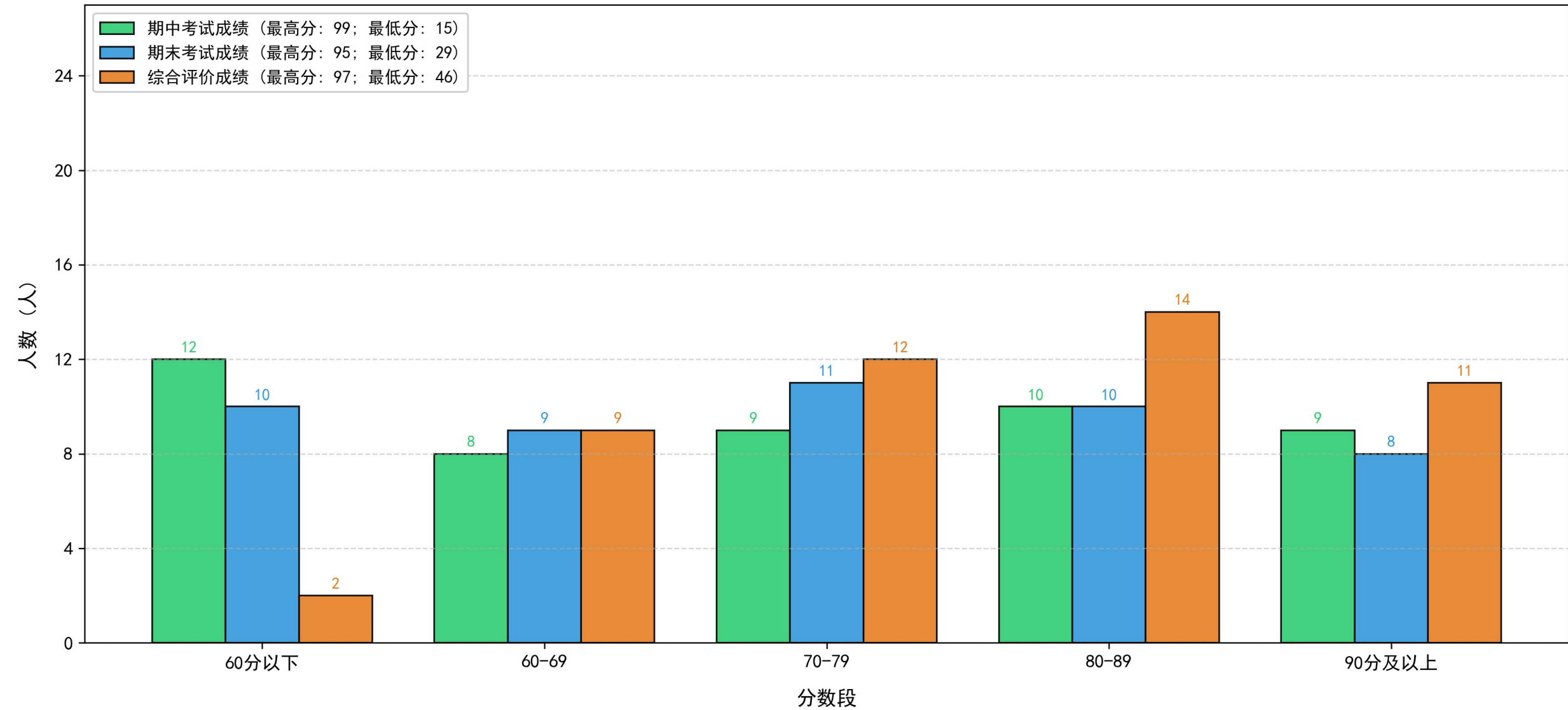
24电22班成绩分布对比图 (总计: 48人)
