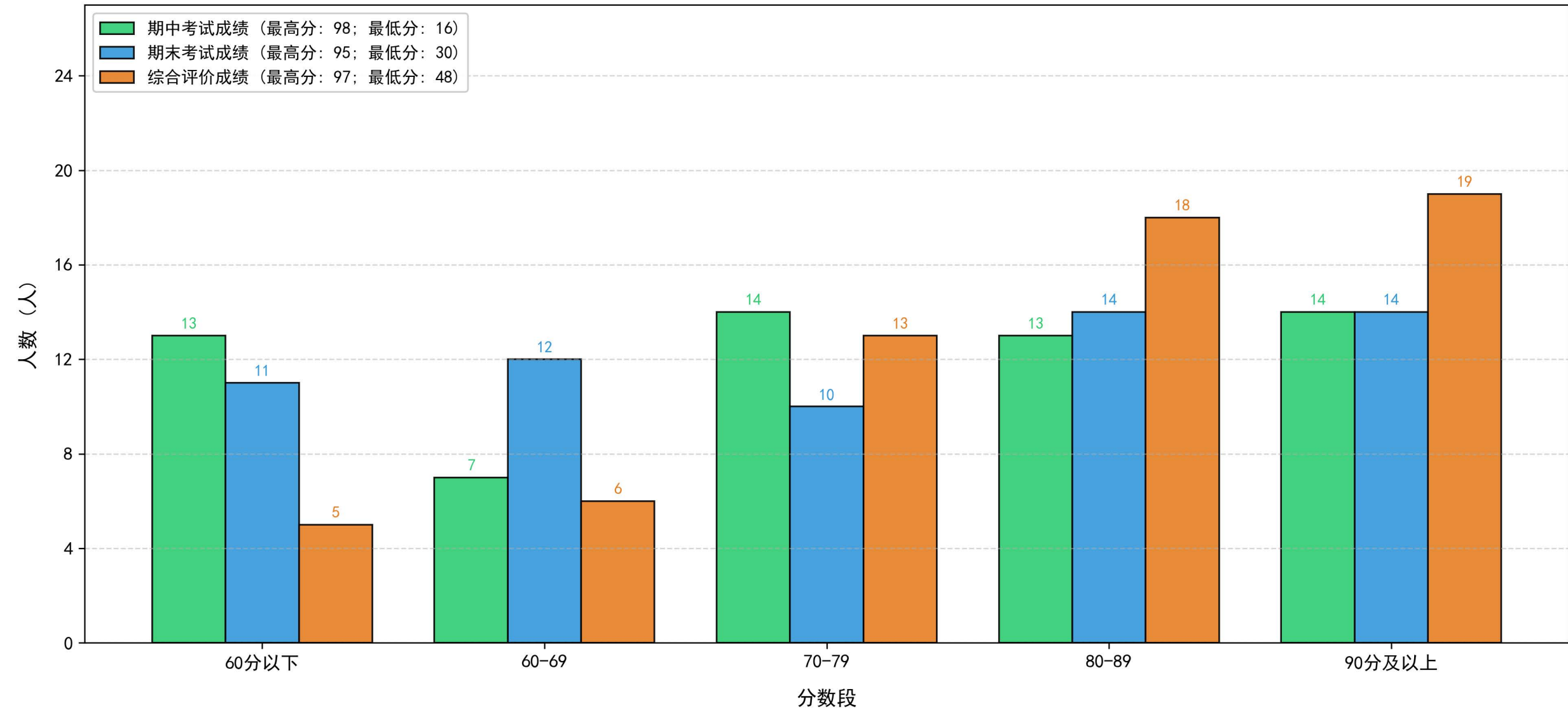
24电12班成绩分布对比图 (总计: 61人)
