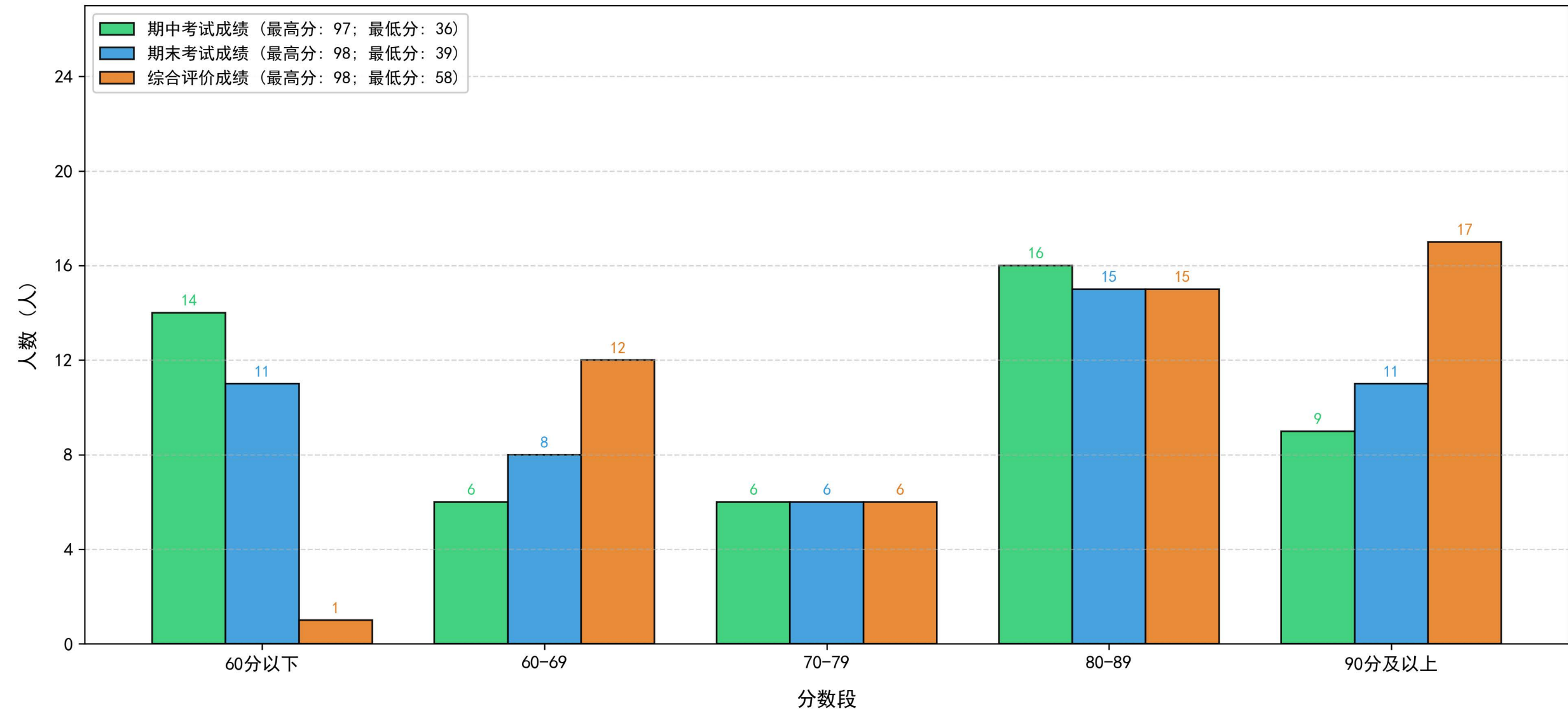
24电21班成绩分布对比图 (总计: 51人)
