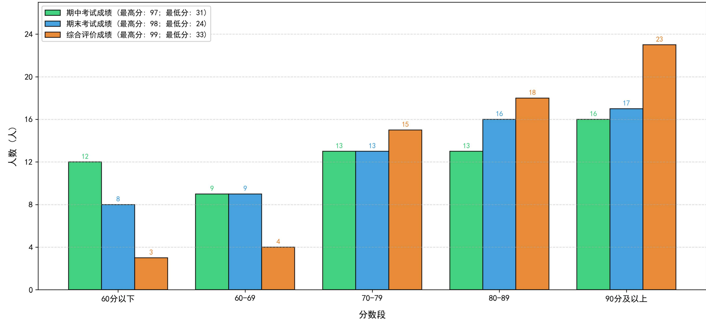
24电11班成绩分布对比图 (总计: 63人)
